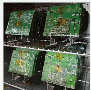
▲ 駐留時間依據測試品表面上風空氣控制示意圖
