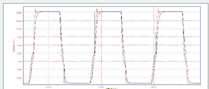
▲ [三箱過常溫衝擊]駐留時間表溫控制實際曲線
