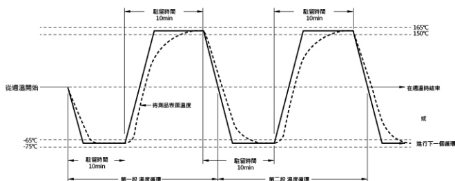
▲ 駐留時間依據測試品表溫控制示意圖
