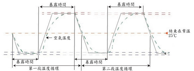
▲ 駐留時間依據測試品表面上風空氣控制示意圖
