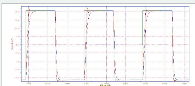
▲ [兩箱高低溫衝擊]駐留時間表溫控制實際曲線
