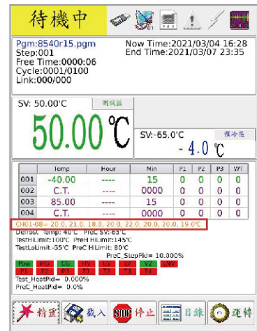
▲ 溫度衝擊過程測試品8軌溫度量測顯示與記錄
